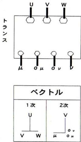
トランス 相3/2 30KVA 50Hz
